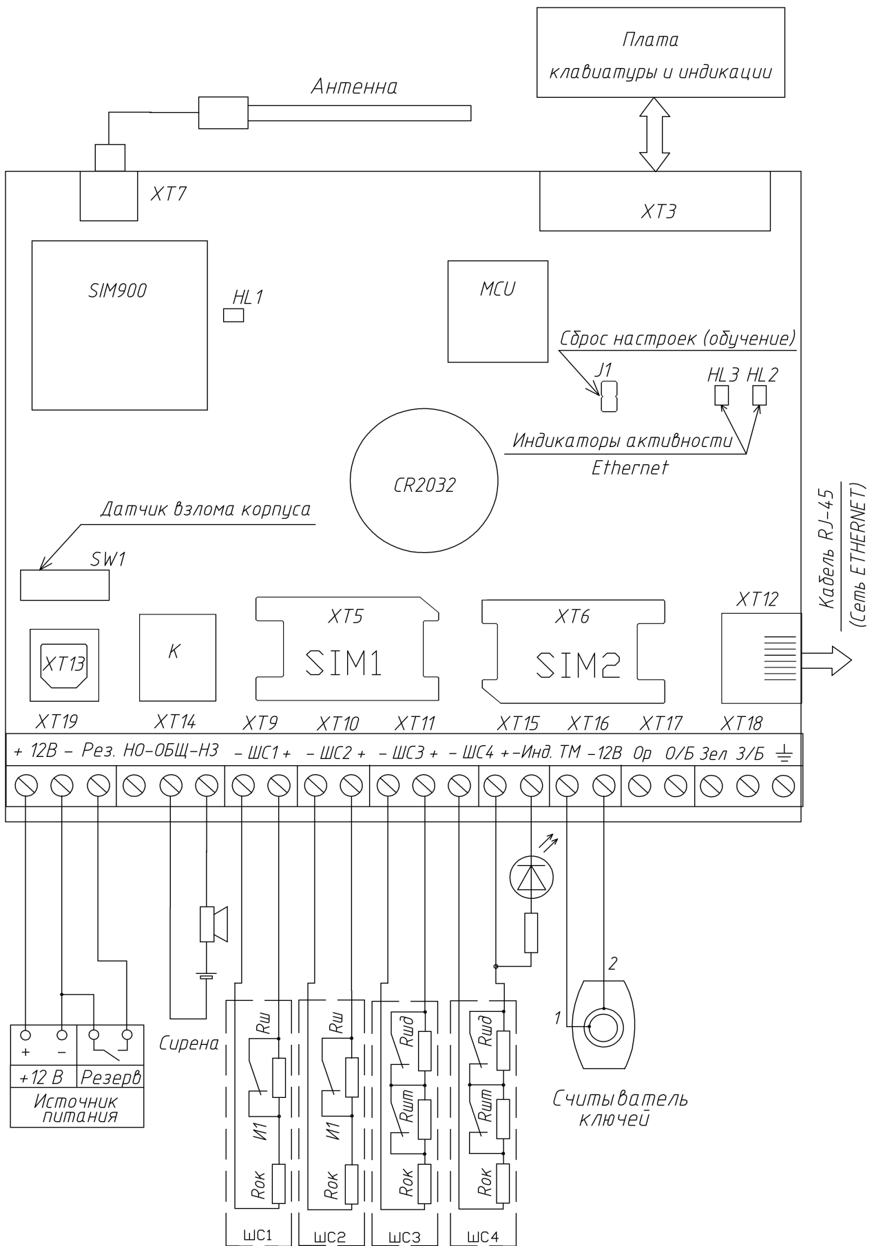
Рис. 5.1 Пример конфигурации прибора
