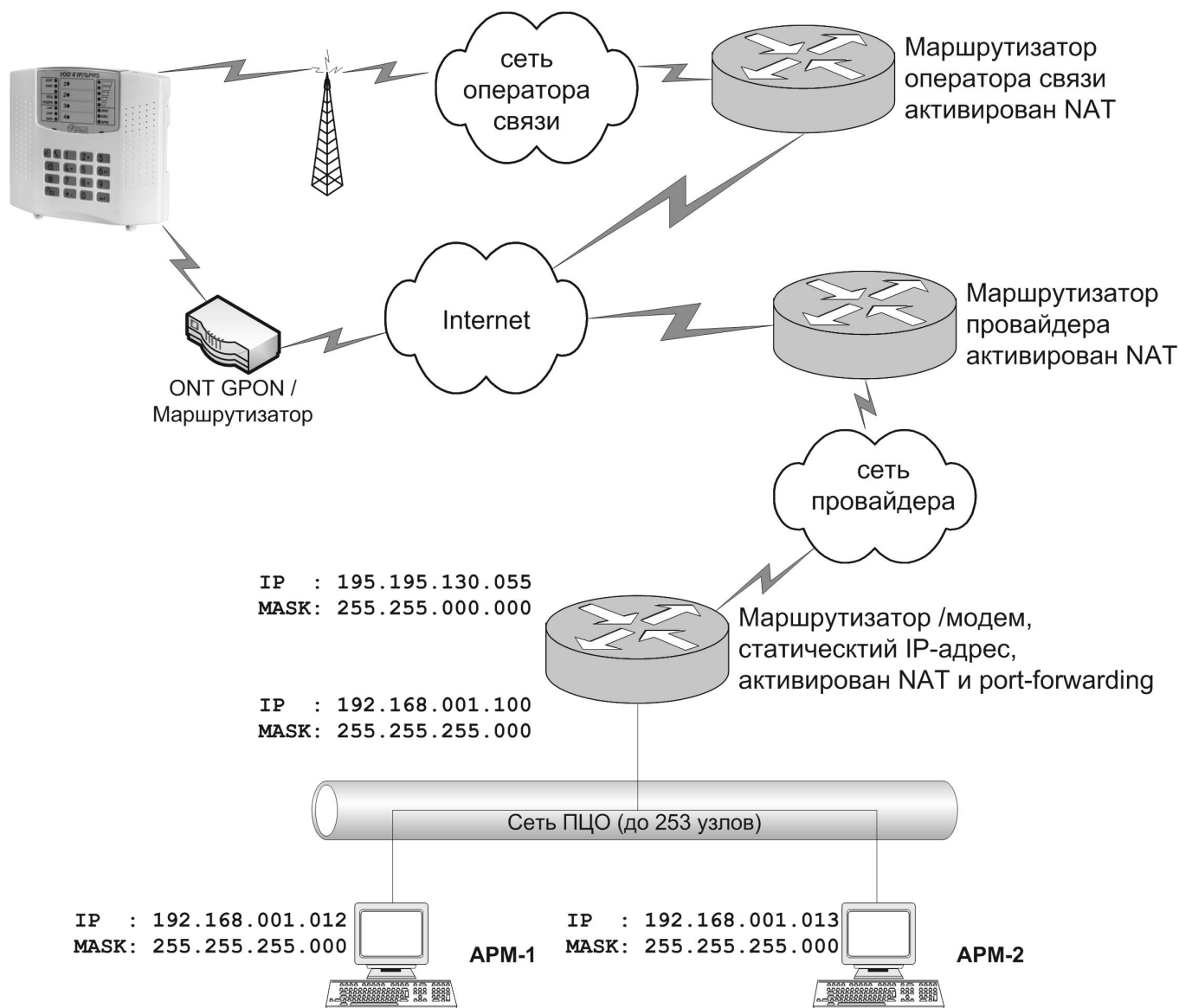
Рис.7.2 Схема работы прибора по каналу Ethernet и GPRS
