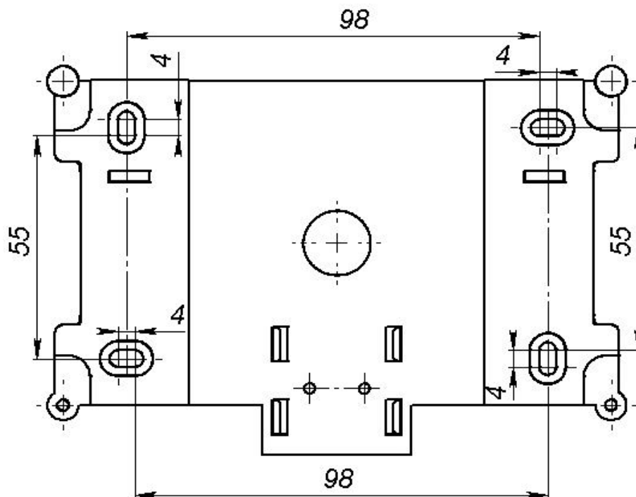
Рис.5.4. Габаритные размеры переходной планки.
